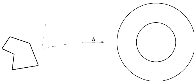
Le dessin correspond au cas 0 < r < R < +\infty
